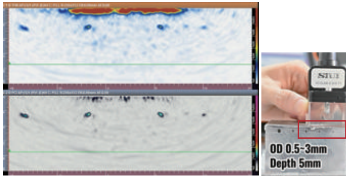
TFM+PCI for holes OD 0.5-3mm
