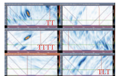
Slag inclusions
