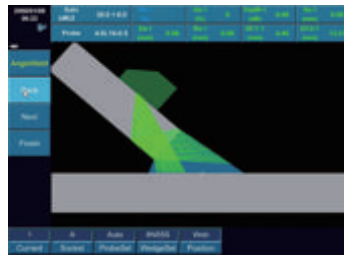
Web Simulation
